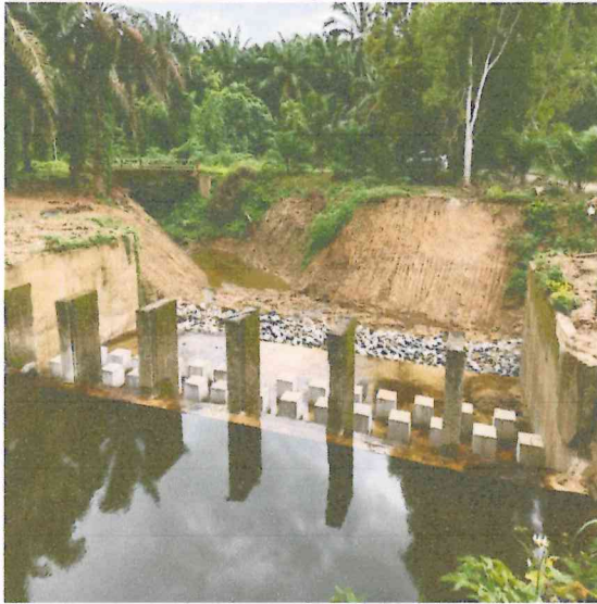
โครงการขุดลอกคลองนาปรัง หมู่ที่ ๑๐ บ้านน้ำหัก ตำบลท่าชะ โดย หน่วยพัฒนาการเคลื่อนที่ ๔๖ สำนักงานพัฒนาภาค ๔ หน่วยบัญชาการทหารพัฒนา
